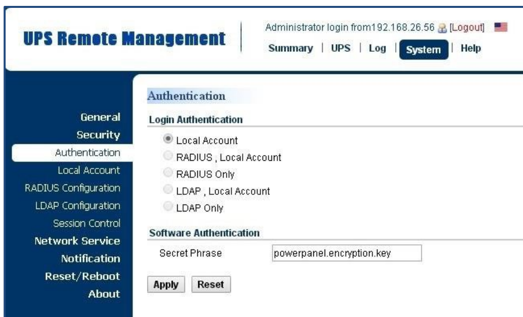
Рисунок 11. Последовательный выбор вкладок «RMCARD System > Authentication» пользовательского интерфейса веб-приложения
