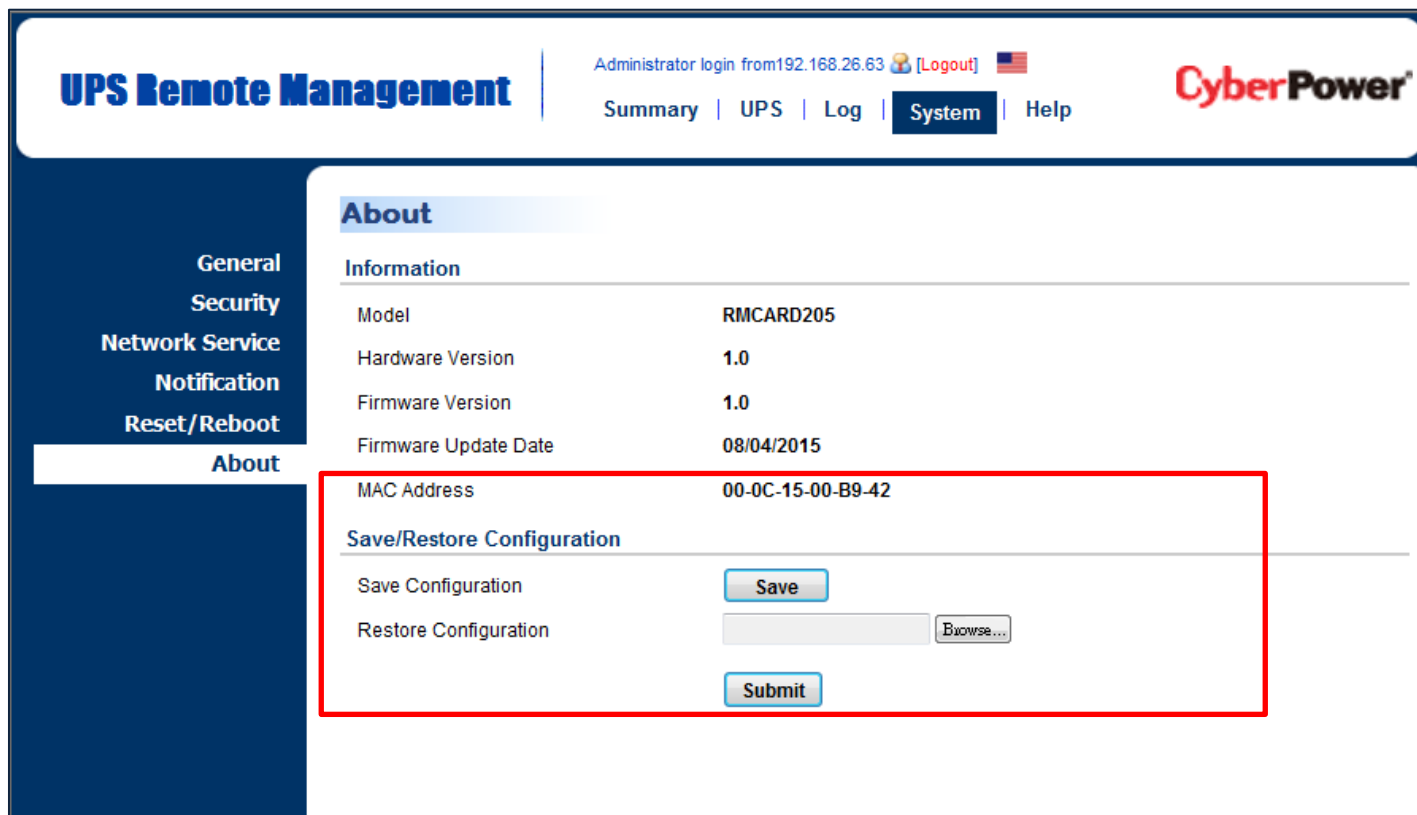
Рисунок 10. Сохранение/восстановление конфигурации в главном окне
