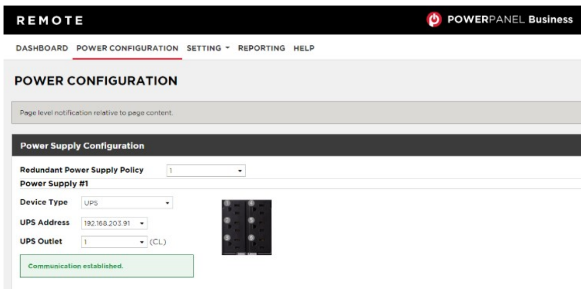
Рисунок 12. Веб-интерфейсе ПО PowerPanel® Business Remote
