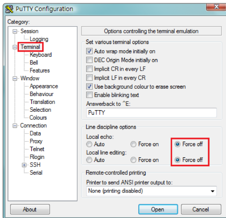
Рисунок 5. Окно конфигурирования PuTTY-клиента.
