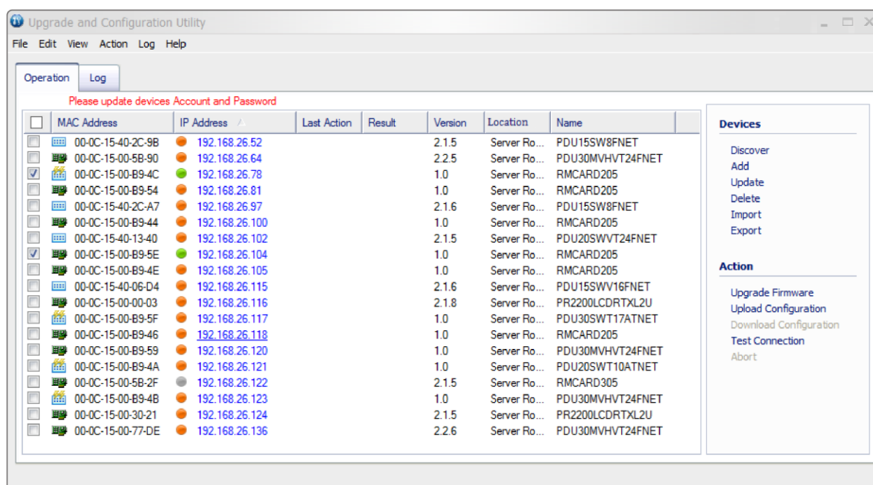
Рисунок 6. Главное окно служебной программы «Upgrade and Configuration Utility»
