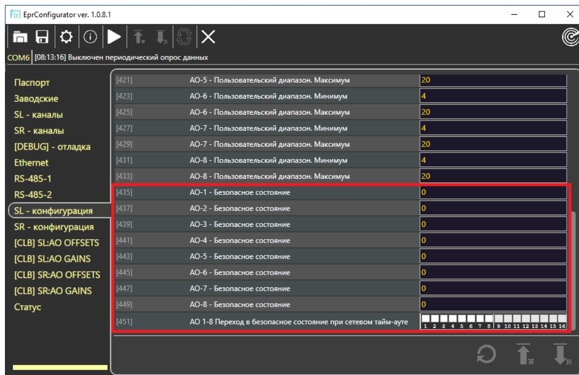
Рисунок 1.6 – Настройка безопасного состояние модуля контроллера Simbol-300 S-300-AO8, S-300-AO16 в СПО EprConfigurator
