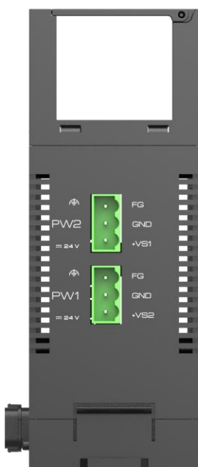
Рисунок 1.4 – Нижняя сторона модуля контроллера Simbol-300 S-300-AO8, S-300-AO16 с разъёмами питания
