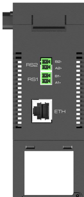
Рисунок 1.3 – Верхняя сторона модуля контроллера Simbol-300 S-300-AO8, S-300-AO16 с разъёмами интерфейсов
