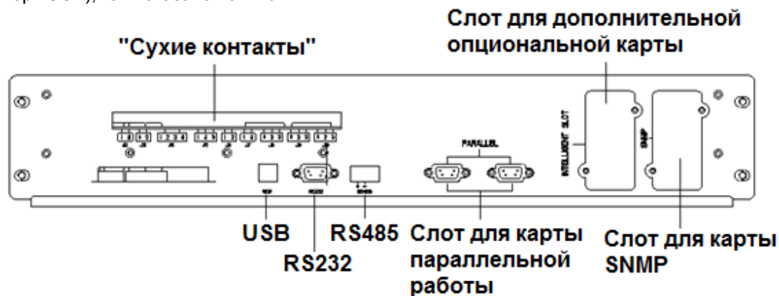
Рис.2-11 Коммуникационные интерфейсы
