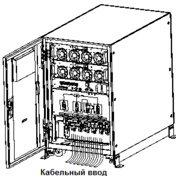
Рис.2-9 Кабельный ввод
