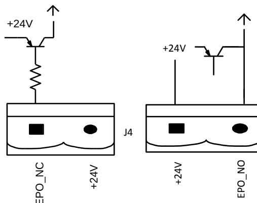
Рис.2-13 Схема разъема системы экстренного отключения (ЕРО)
