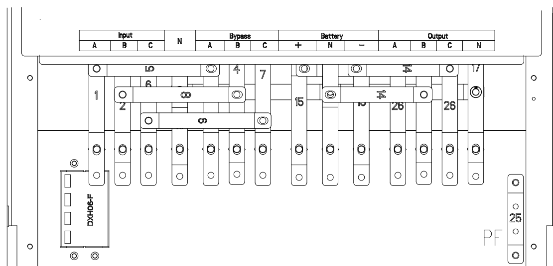
Рис.2-10 Клеммная колодка
