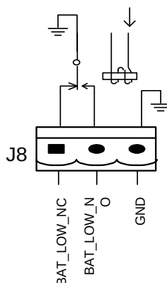
Рис.2-16 Схема разъема сигнализации о низком уровне заряда батарей
