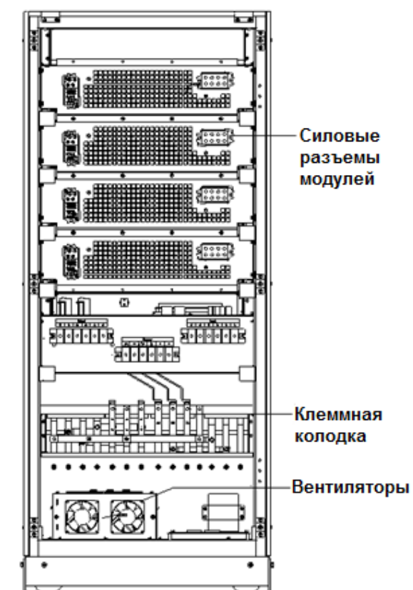
Рис. 1-11 Компонировка ИБП 80-120кВА Вид сзади
