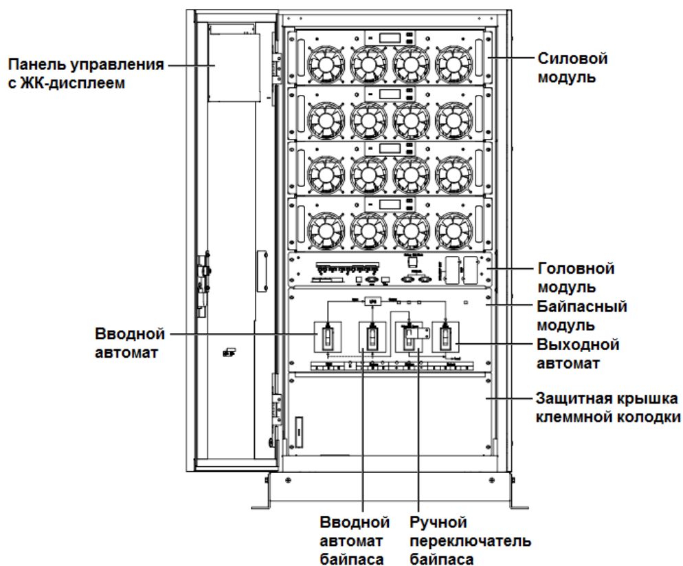
Рис.1-10 Компонировка ИБП 80-120кВА Вид спереди
