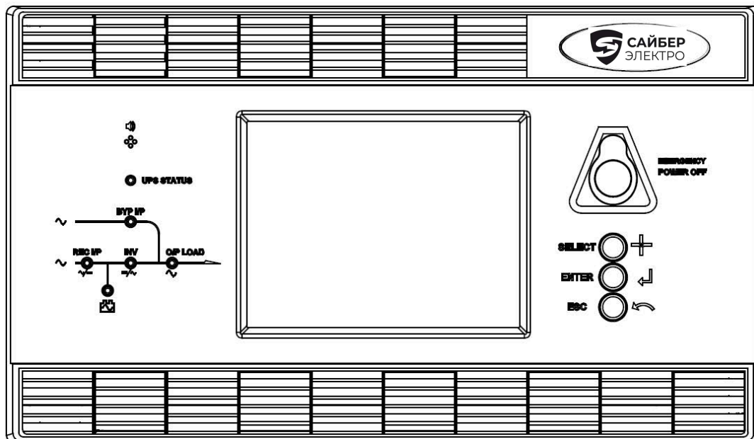
Рис.3-1 Панель оператора
