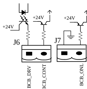
Рис.2-15 Схема разъемов BCB
