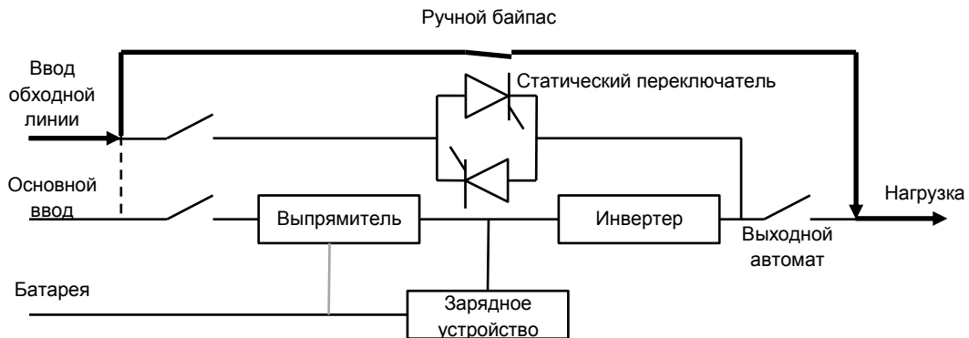
Рис.1-6 Режим обслуживания
