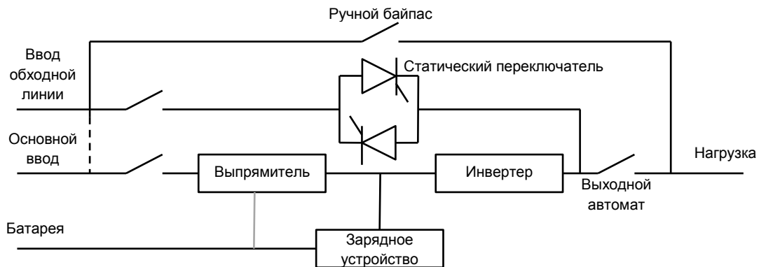
Рис.1-1 Схема ИБП
