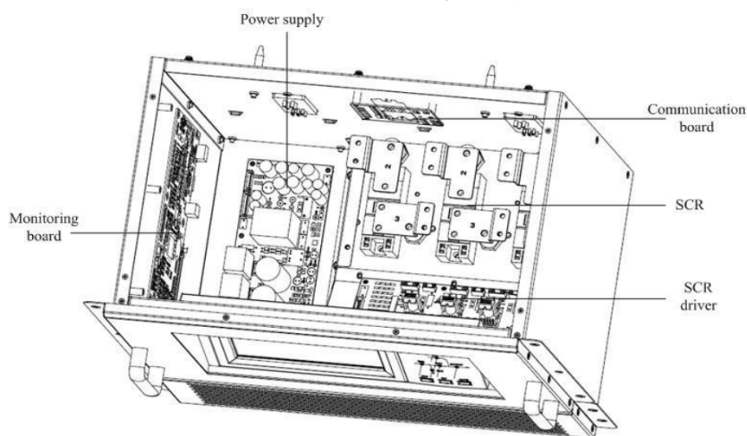
Рис. 3-10-1 Байпасный модуль 60/90kVA.
