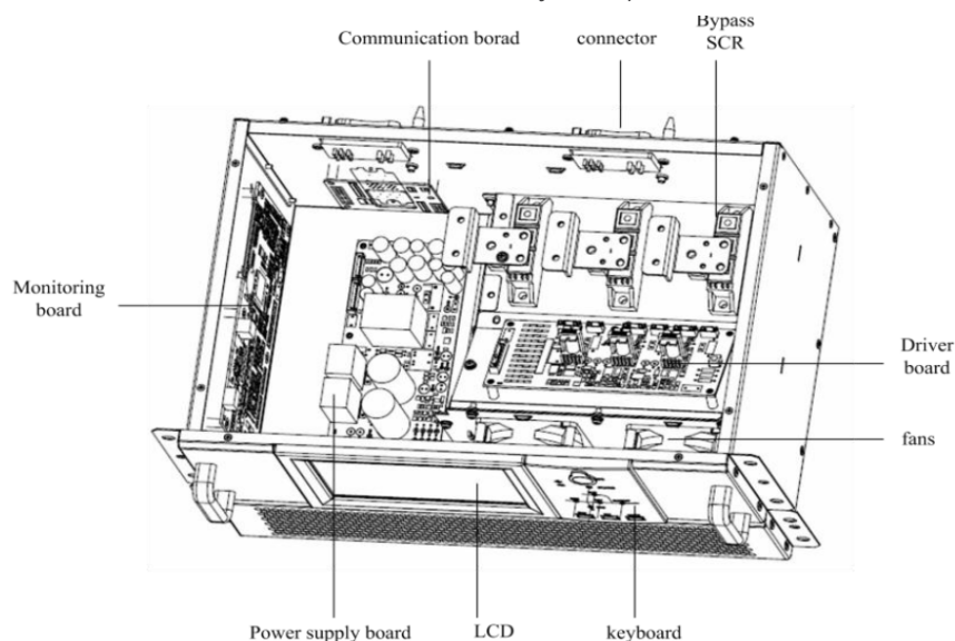
Рис. 3-10-1 Байпасный модуль 30/45kVA.
