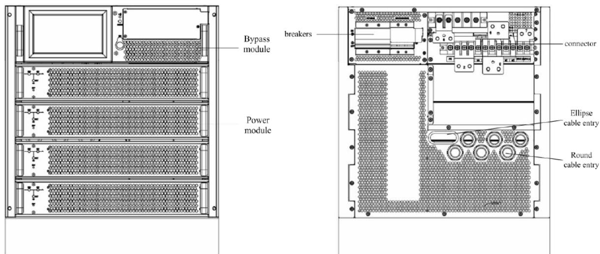
Рис. 1-2 Кабинет на 4 модуля
