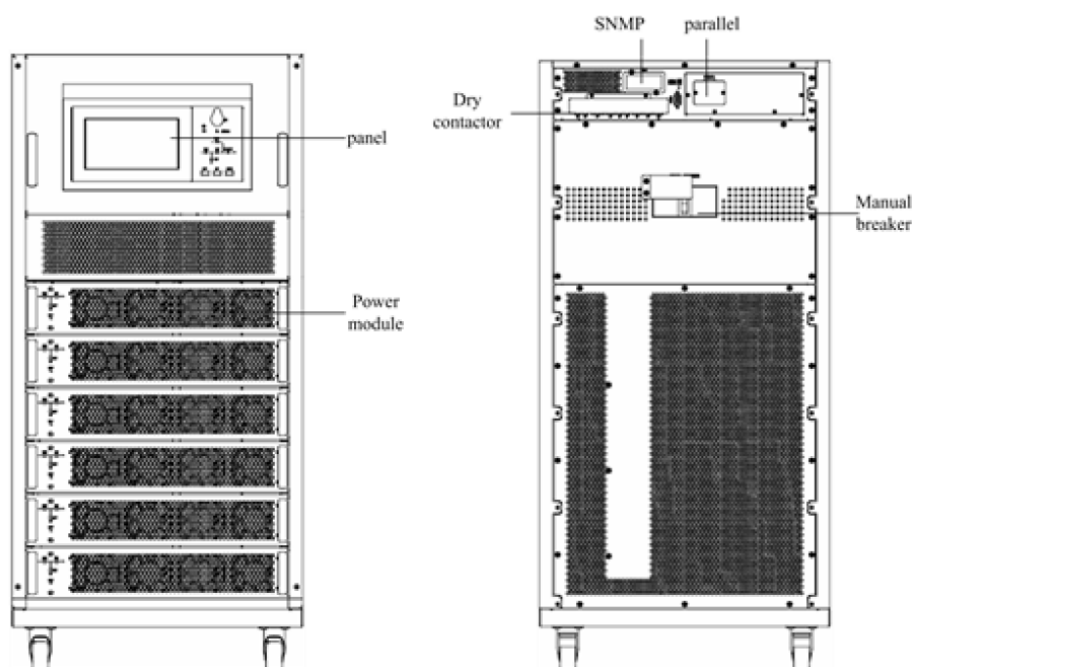
Рис. 1-1 Кабинет на 6 модулей
