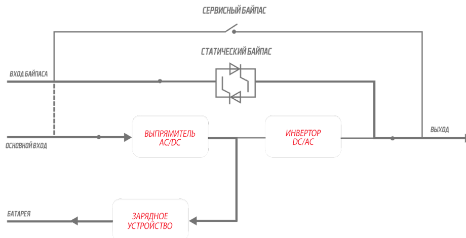
Рис. 2-7 ECO режим
