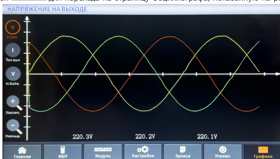
Рис. 4-11 Экран осциллографа
