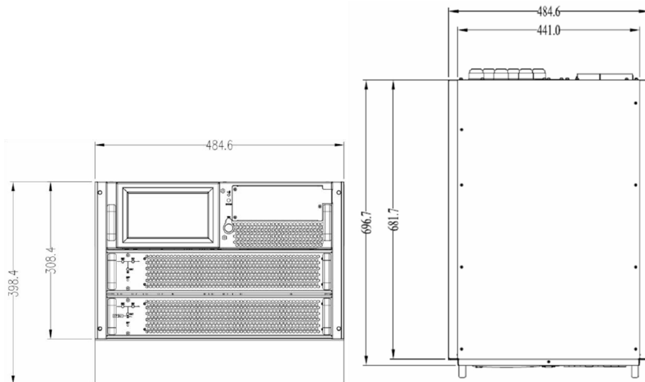
Рис. 3-2-2 Габариты силового шкафа на 2 модуля
