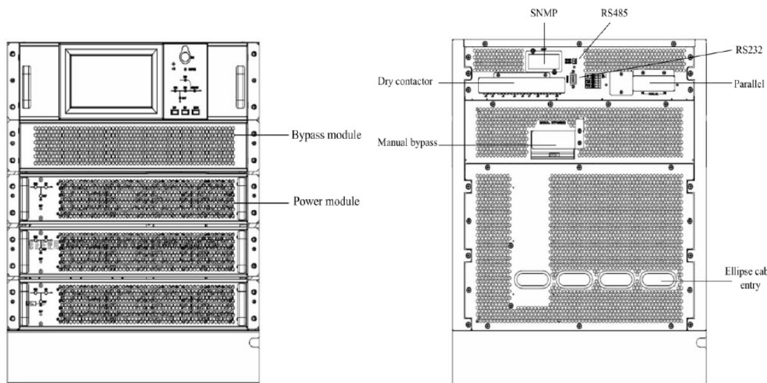
Рис. 1-3 Кабинет на 3 модуля
