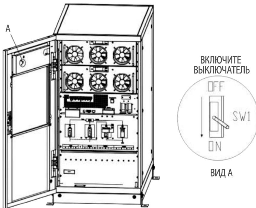
Рис. 5-2. Переключатель на передней панели
