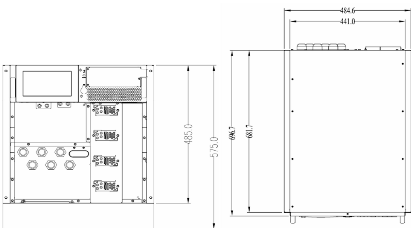
Рис. 3-2-1 Габариты силового шкафа на 4 модуля
