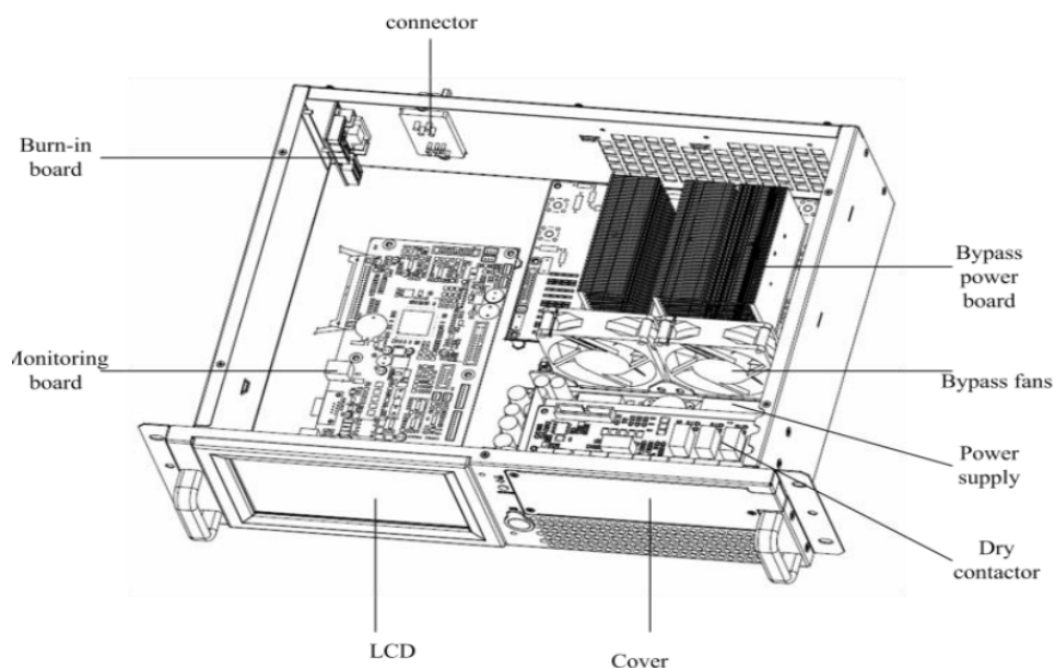
Рис. 3-10 Байпасный модуль 20/40kVA.
