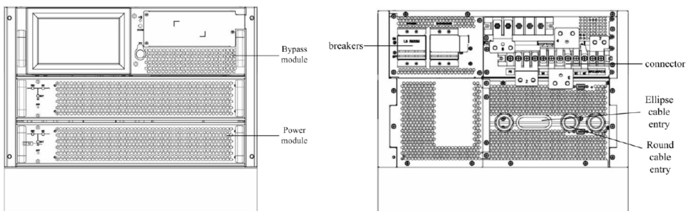
Рис. 1-4 Кабинет на 2 модуля
