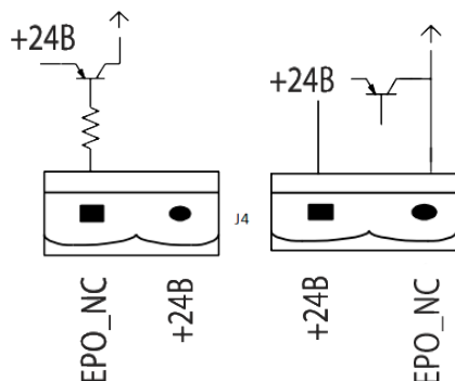
Рис.3-14 Схема разъема системы экстренного отключения (ЕРО)
