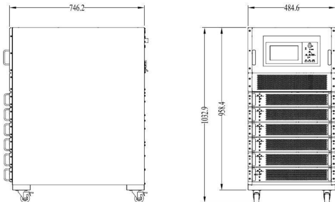
Рис. 3.1 Габариты силового шкафа на 6 модулей
