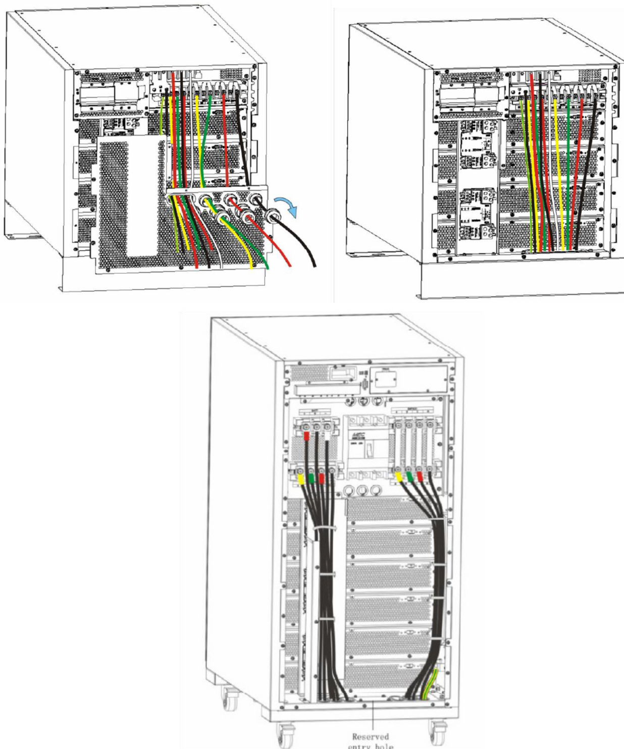
Рис. 3-9 Кабельный ввод
