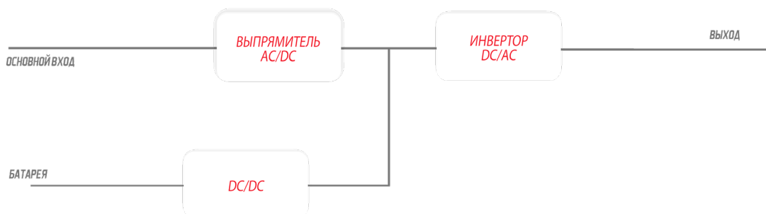
Рис. 2-1 Конфигурация ИБП
