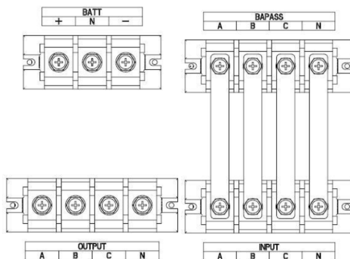
Рис. 3-11-2 Клемная колодка ИБП 60/90kVA.
