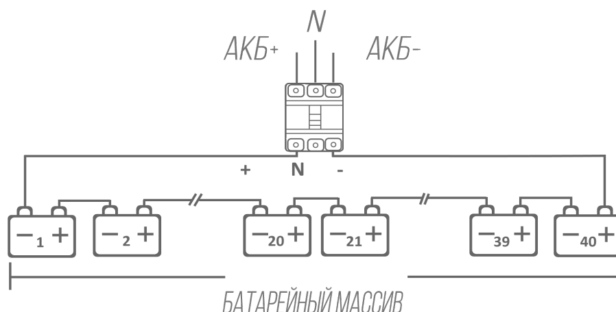
Рис. 3-8 Схема подключения батарей
