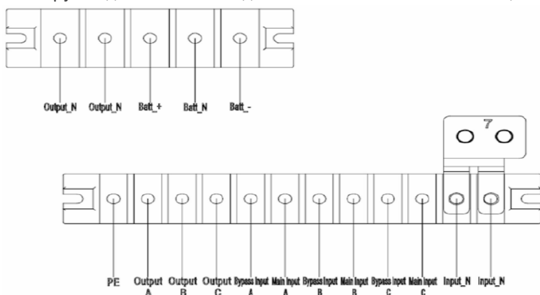
Рис. 3-11-1 Клемная колодка ИБП 20/40kVA.
