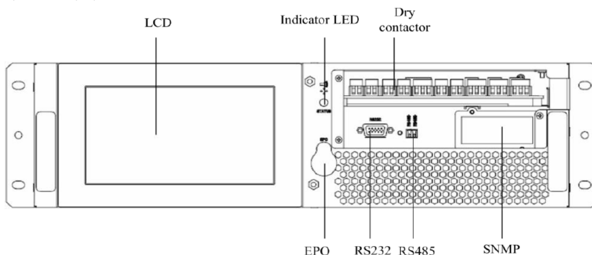
Рис.3-12-1 20/40kVA байпасный модуль
