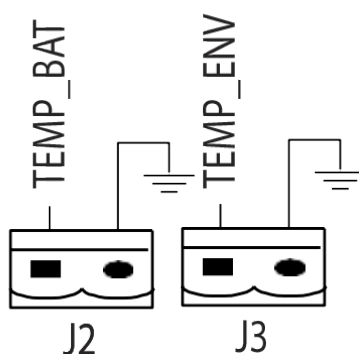
Рис.3-13 Схема разъемов J2 и J3 для датчиков температуры
