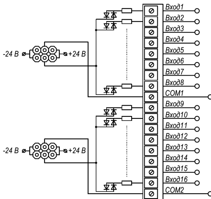
Рисунок 1.4 – Установка джамперов для различных схем питания входных каналов
