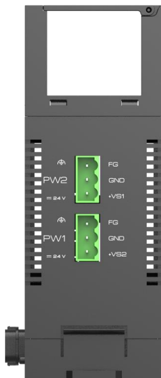
Рисунок 1.4 – Нижняя сторона модуля контроллера Simbol-300 S-300- DI16, S-300-DI32 с разъёмами питания
