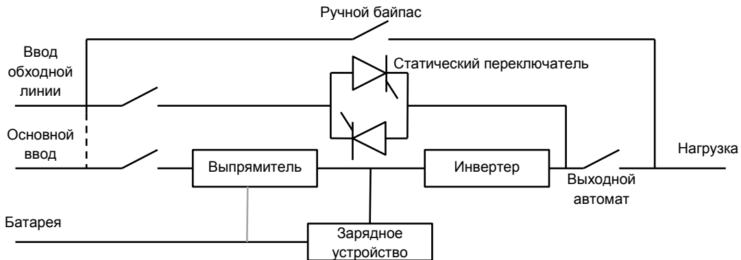
Рис.1-1 Схема ИБП
