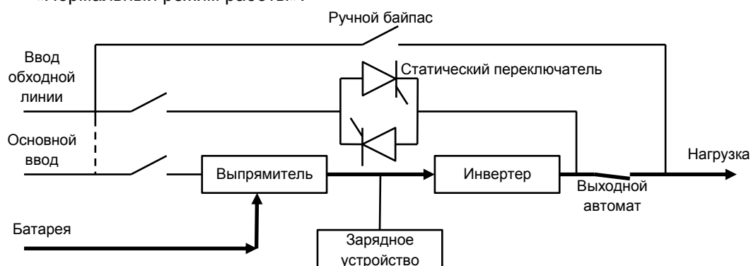
Рис.1-4 Режим работы от батарей
