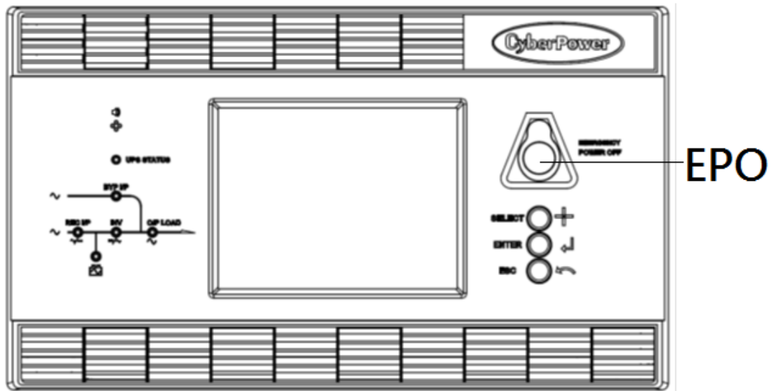
Рис .4-5 Кнопка экстренного выключения ИБП (ЕРО)
