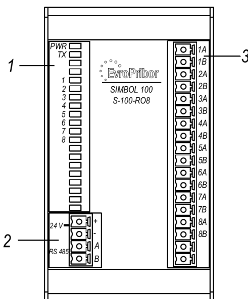
Рисунок 1.2 – Лицевая панель модуля релейных выходов S-100-RO8
