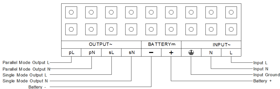
Рис.2 Схема подключения входных и выходных клемм
