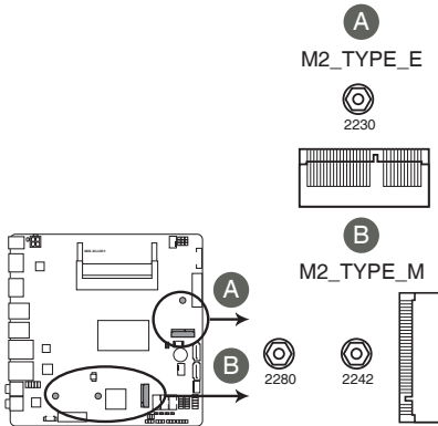
MIX-KLUD1 M.2 sockets
