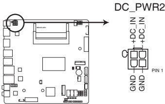
MIX-KLUD1 DCIN power connector
