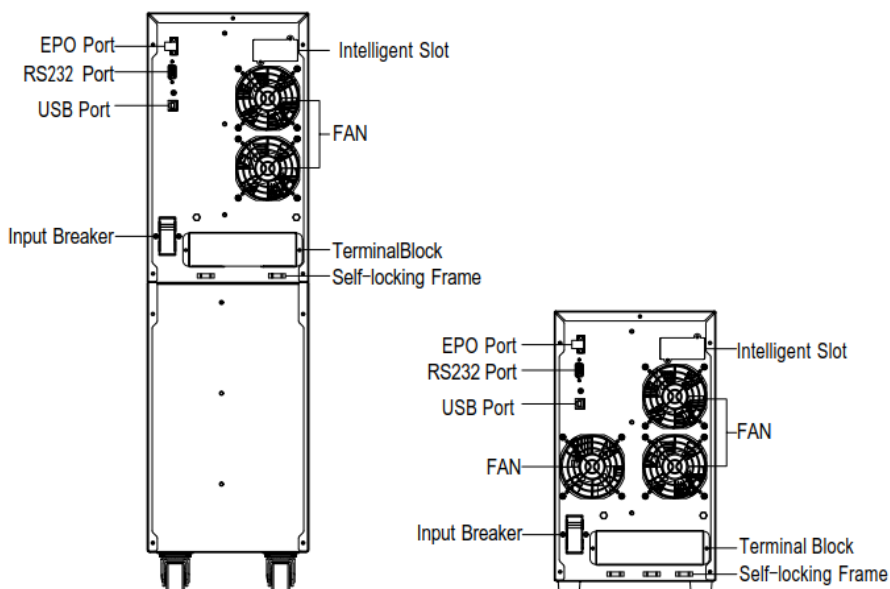
ЭКСПЕРТ-6000/ЭКСПЕРТ-10000 ЭКСПЕРТ-6000XL/ЭКСПЕРТ-10000XL Рис.3-1 ЗАДНЕЙ ПАНЕЛИ ИБП
