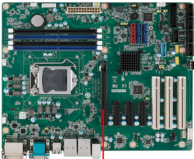
PCIe x16_1
