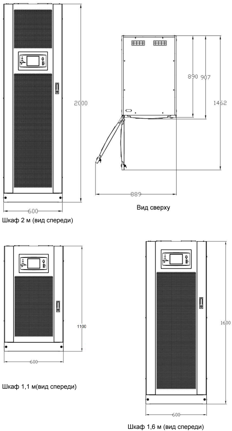
Рис. 1-22. ИБП, вид спереди (размеры приводятся в мм)
