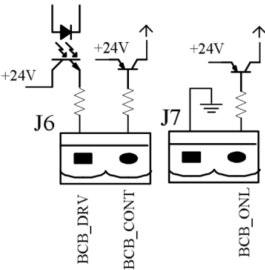
Рис. 1-16. Интерфейс BCB
