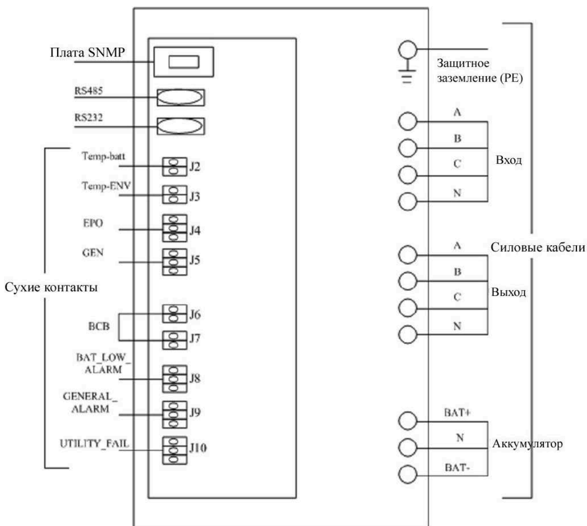
Рис. 1-21. Схема установки
