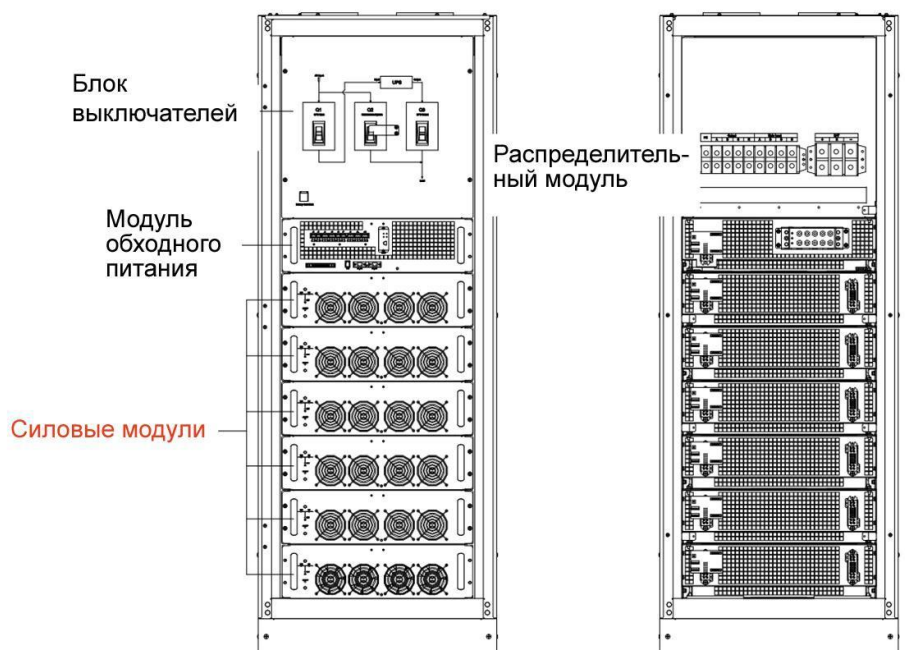
Шкаф 1,6 м (вид спереди)
