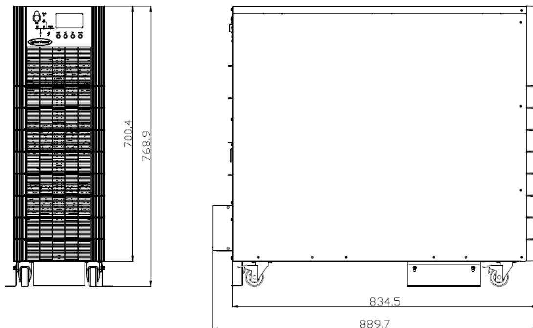
Рис.2-3 Габариты ИБП 40кВА (ед. изм.: мм)
