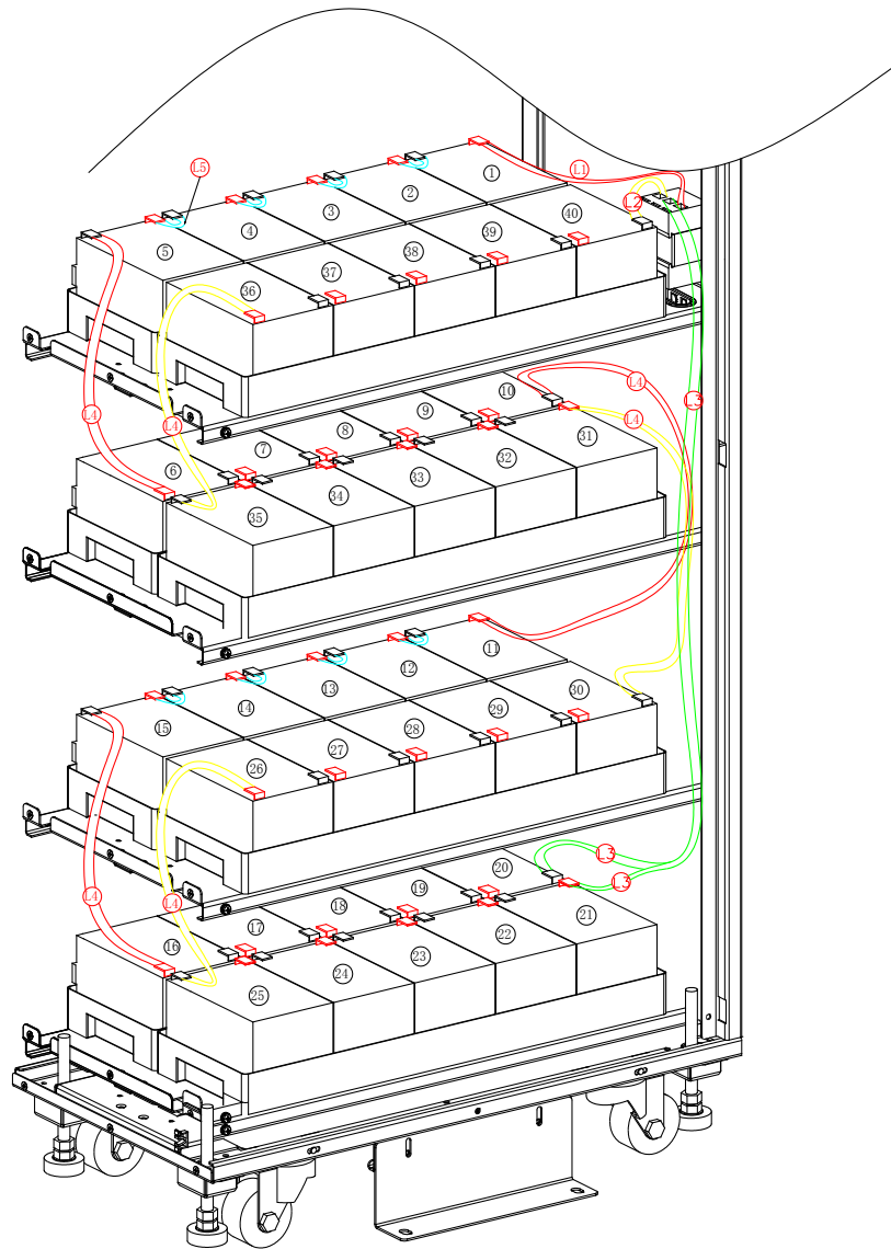
Рис.5-2-1 Соединение батарей
