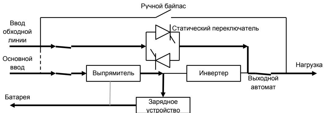
Рис.1-6 Экономичный режим
