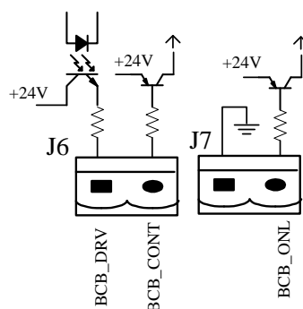
Рис.2-18 Схема разъемов ВСВ
