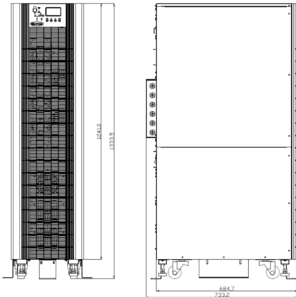
Рис.2-2-2 Габариты ИБП 20/30кВА со встроенными батареями (ед. изм.: мм)
