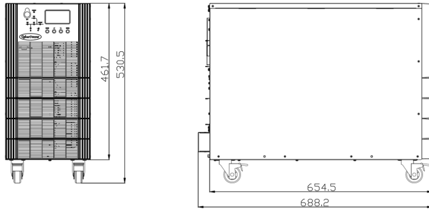
Рис.2-1-1 Габариты ИБП 10/15кВА без встроенных батарей (ед. изм.: мм)
