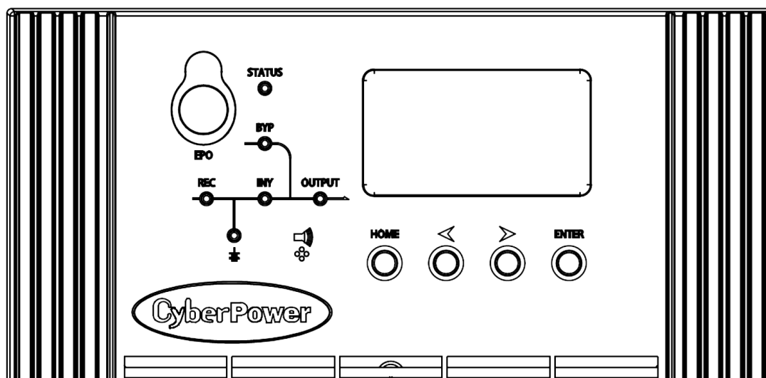
Рис.3-1 Панель оператора
