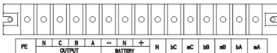
Рис.2-11 Клеммная колодка на ИБП 10/15кВА
