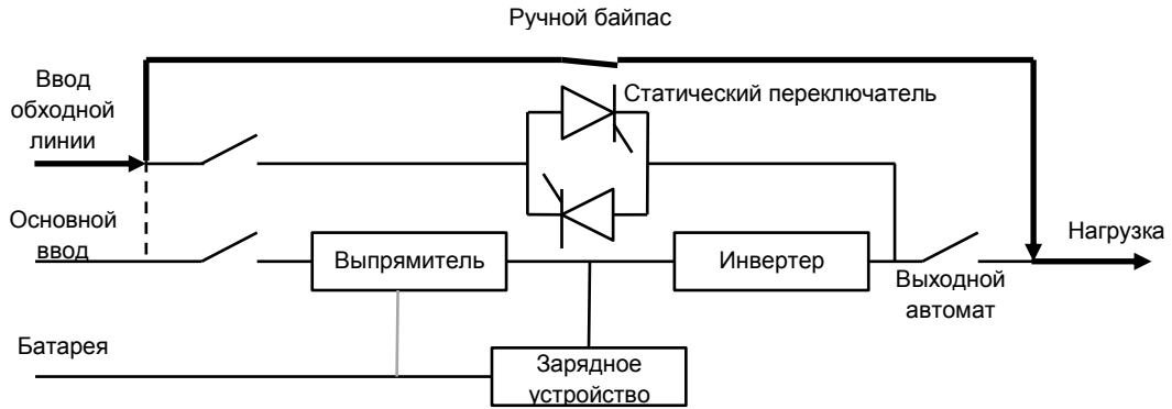
Рис.1-5 Режим обслуживания
