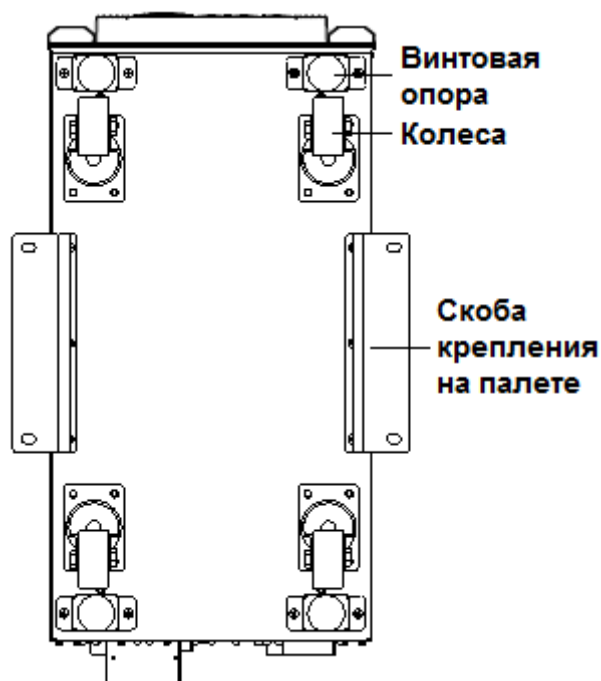
Рис.2-8 Винтовые опоры и колеса (вид снизу)
