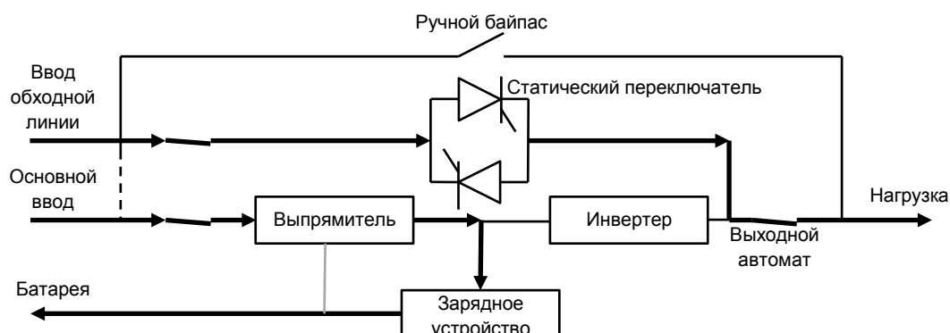
Рис.1-4 Режим обходной линии
