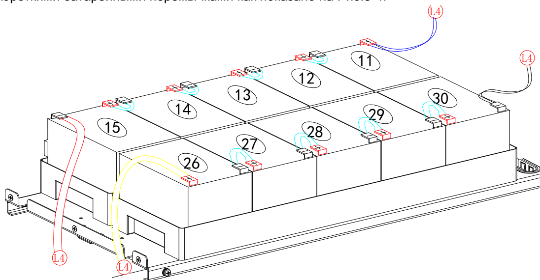
Рис.5-2-4 Соединение батарей. Уровень 3
