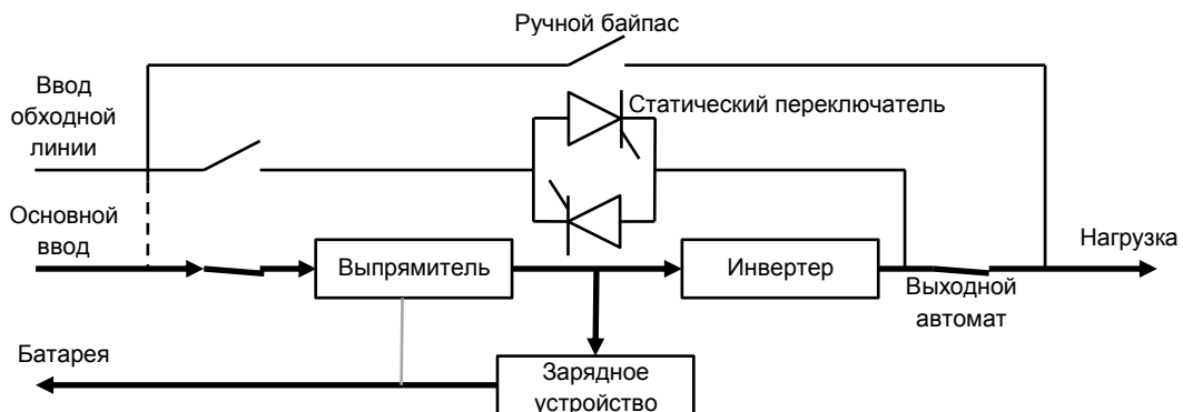
Рис.1-2 Нормальный режим работы
