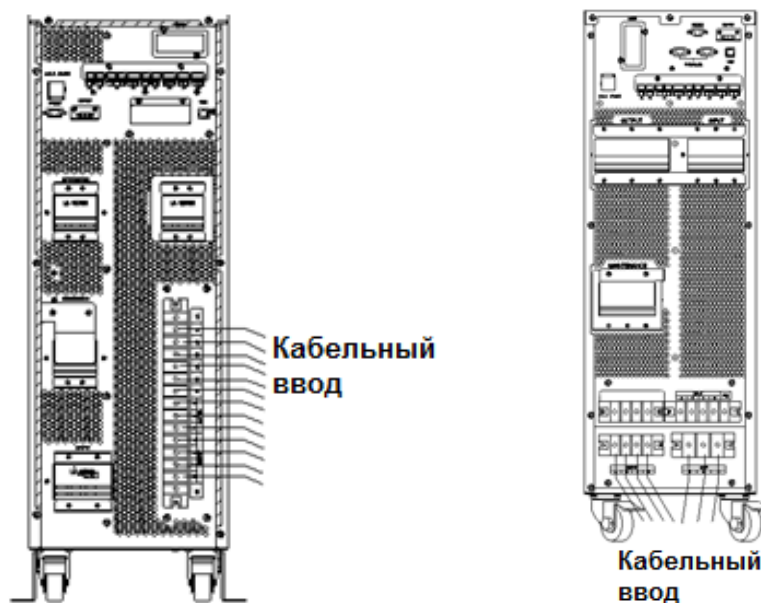
Рис.2-10 Кабельный ввод
