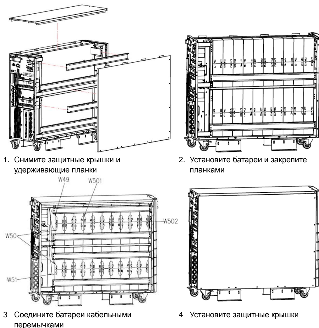
Рис.5-1 Установка батарей
