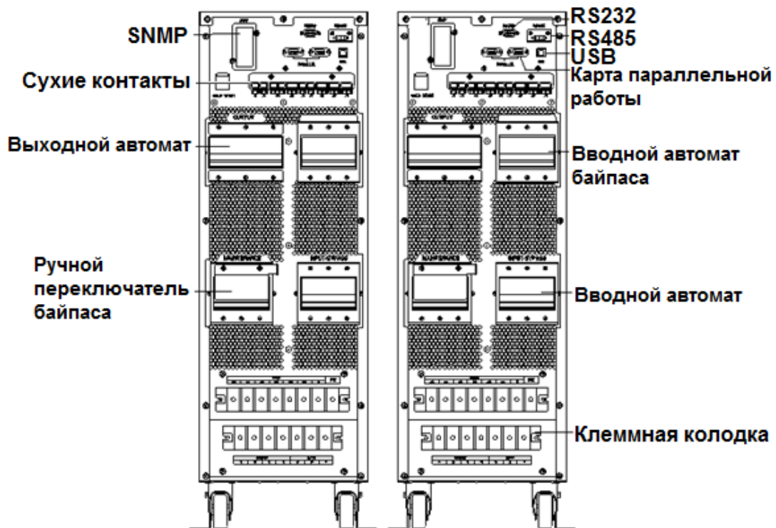
Рис.1-13 Компоновка ИБП 40кВА, вид сзади
