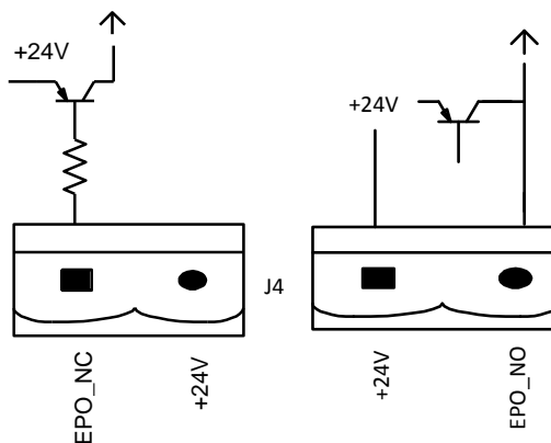
Рис.2-16 Схема разъема системы экстренного отключения (EPO)
