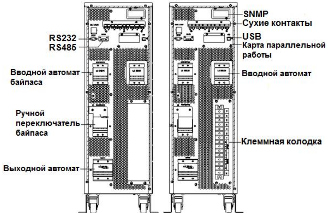
Рис.1-12 Компоновка ИБП 20/30кВА, вид сзади
