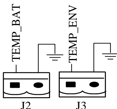
Рис.2-15 Схема разъемов J2 и J3 для датчиков температуры
