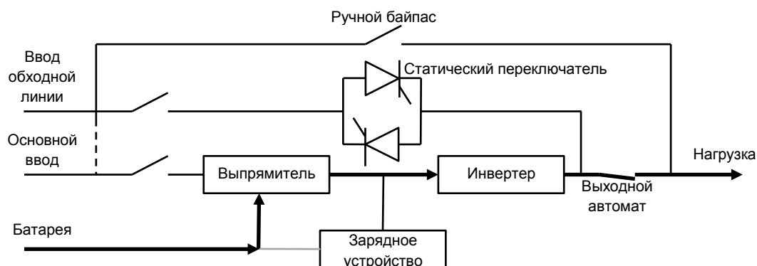
Рис.1-3 Режим работы от батарей
