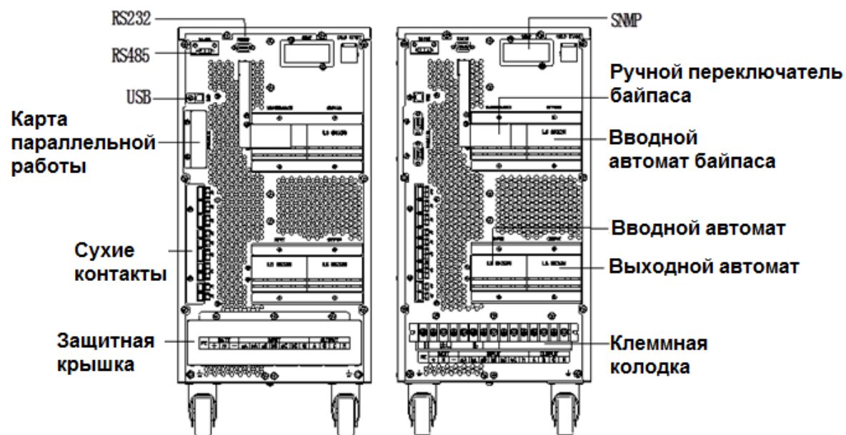
Рис.1-11 Компоновка ИБП 10/15кВА, вид сзади
