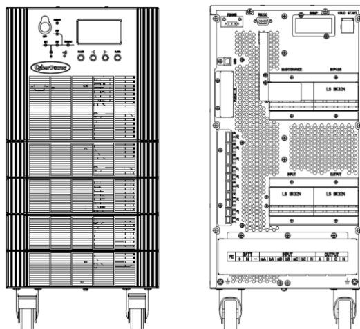
Рис.1-7 Внешний вид ИБП 10/15кВА
