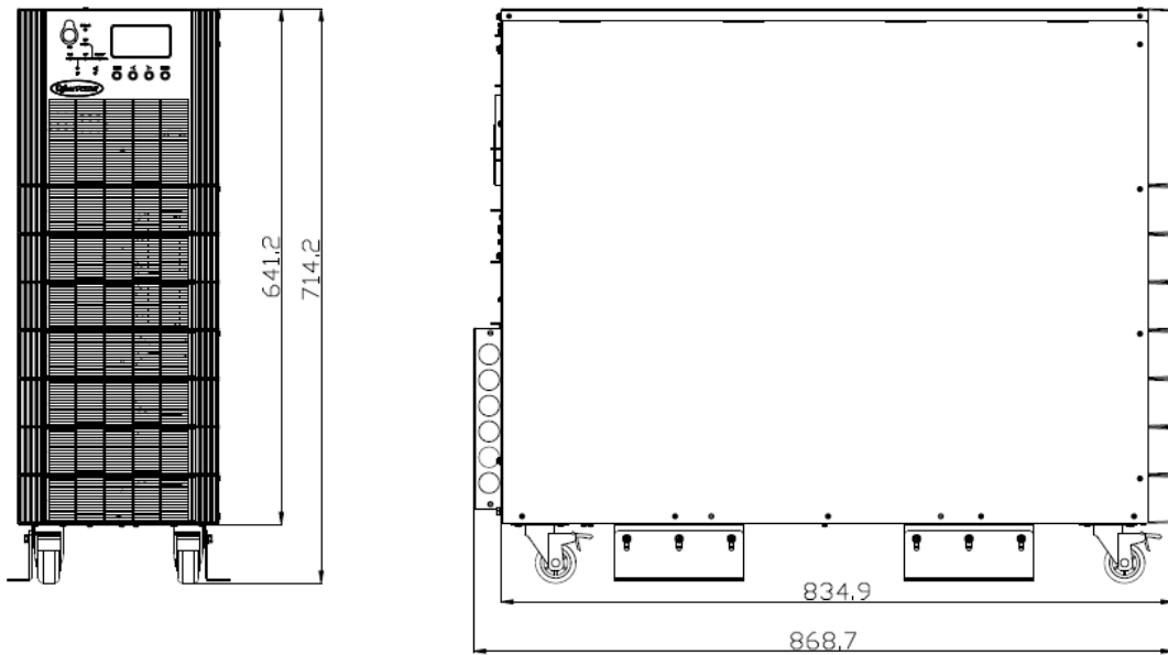
Рис.2-1-2 Габариты ИБП 10/15кВА со встроенными батареями (ед. изм.: мм)
