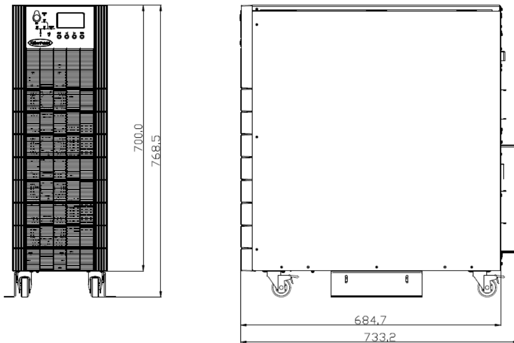
Рис.2-2-1 Габариты ИБП 20/30кВА без встроенных батарей (ед. изм.: мм)
